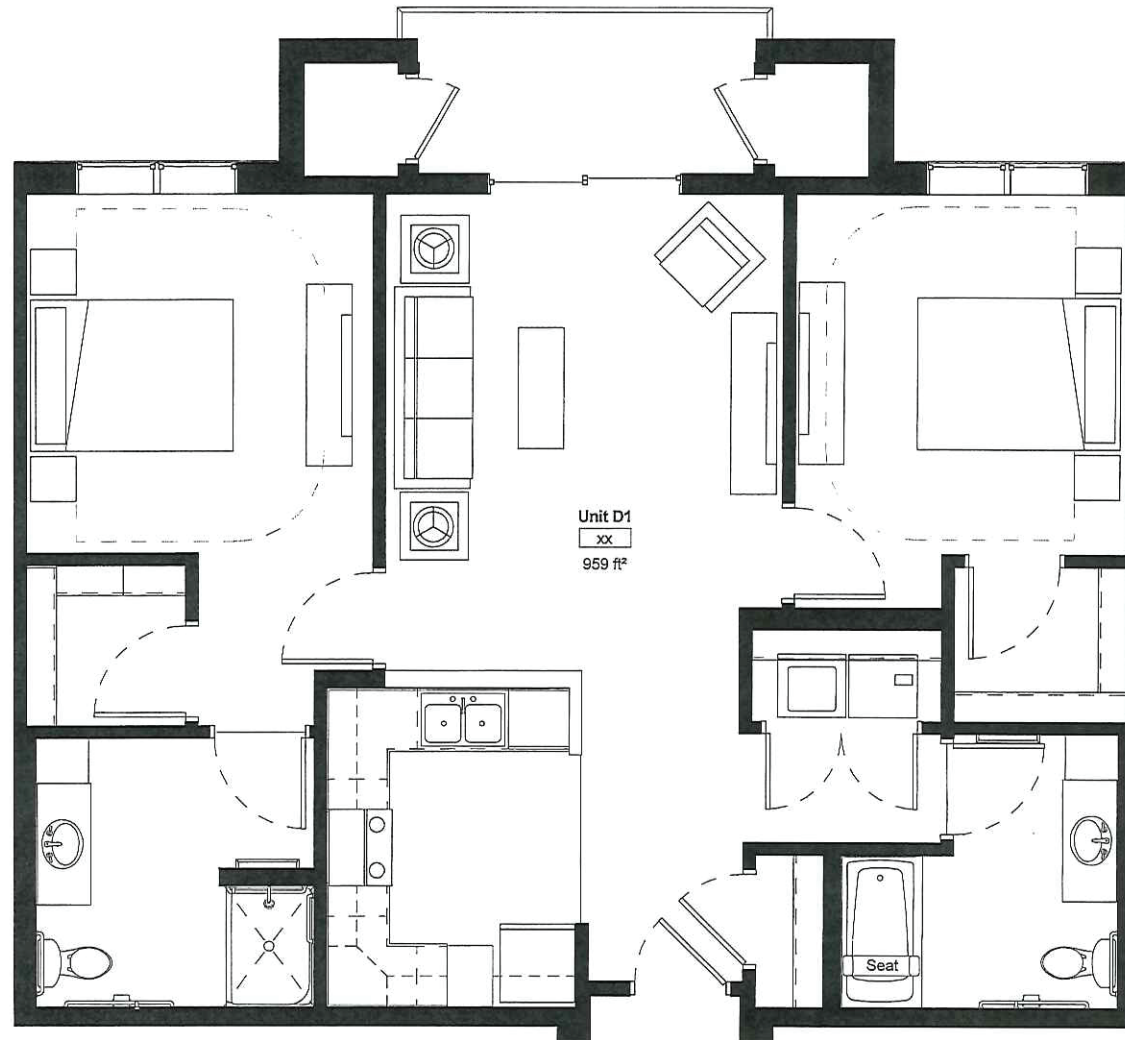
① Unit Plan - D1 1/4" = 1'-0"
